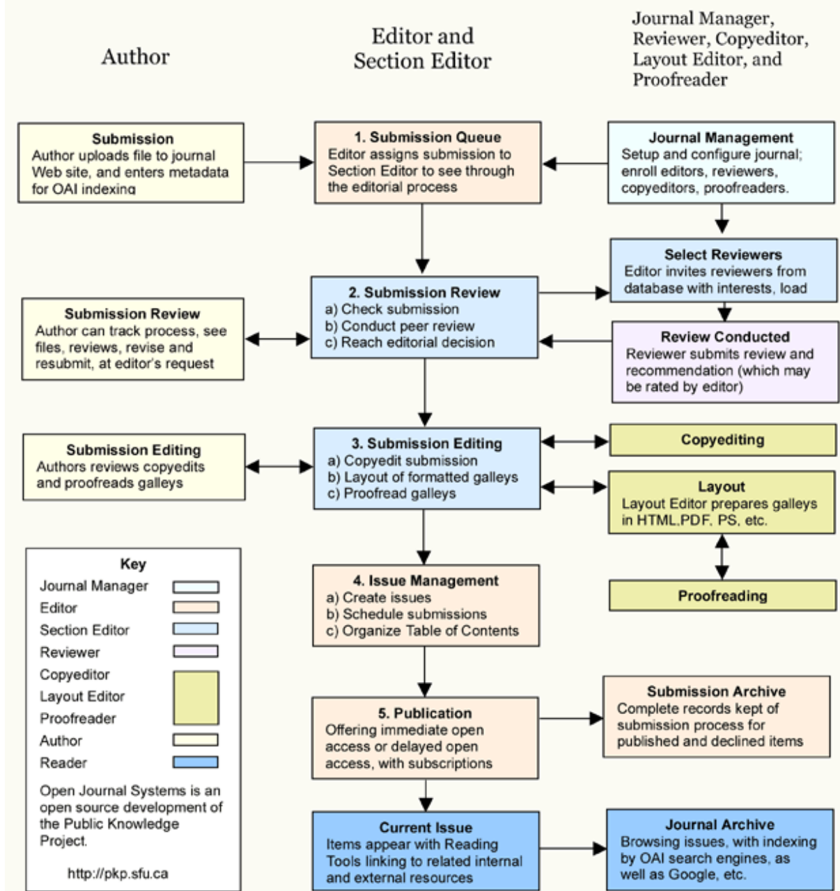
Schéma procesu editace a publikování Open Journal Systems 2.4.2.0 .
