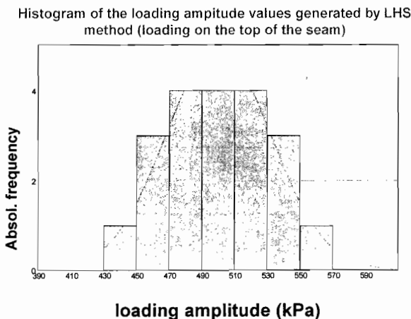
Obr.3 Histogram amplitud generovaných metodou LHS pro zatížení iniciované na hlavě sloje
