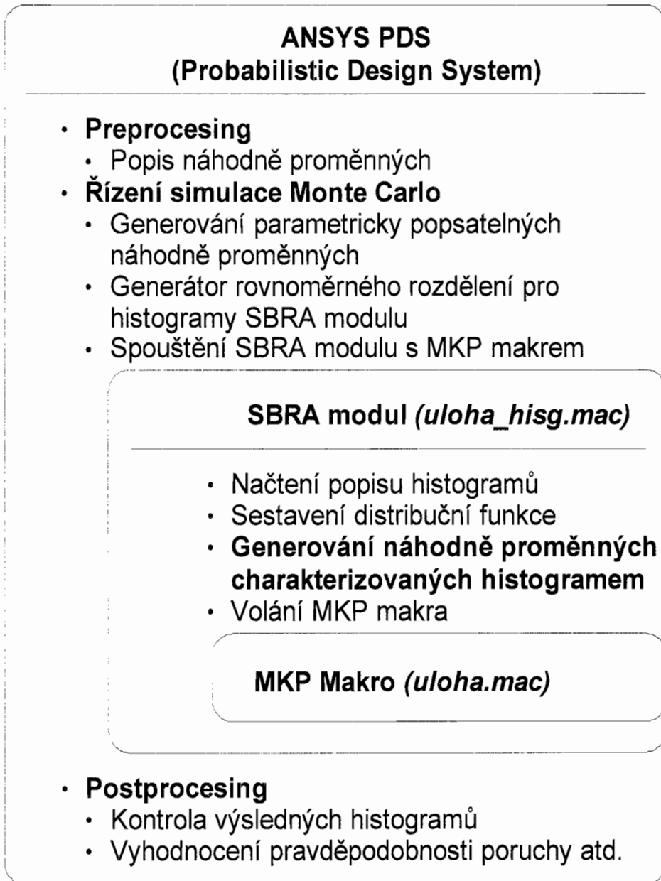
Obr.1 SBRA modul v rámci stochastického modulu MKP programu ANSYS
