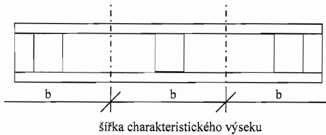
Obr.1 Charakteristický výsek konstrukce se systematickými tepelnými mosty
